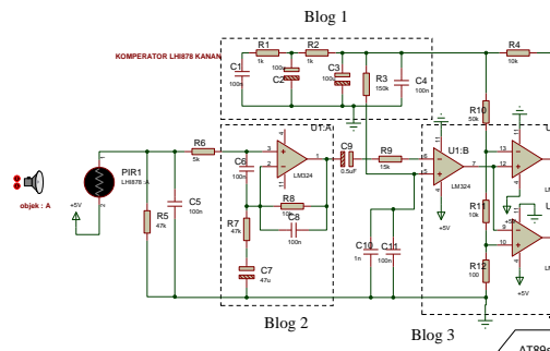
Gambar 4. Komparator Sensor PIR
