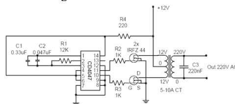
Gambar 3. Rangkaian perancangan
