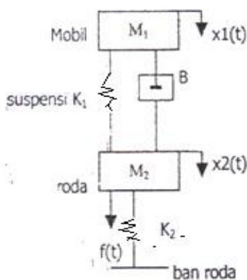
Gambar 1. Sistem Suspensi Kendaraan
