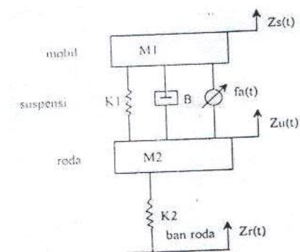
Gambar 2. Sistem Suspensi Aktif Kendaraan
